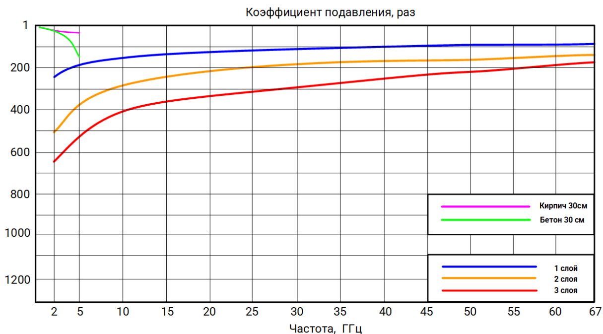
Рисунок 2 – Коэффициент подавления СВЧ-энергии волны типа Н 10 в волноводных сечениях в размах для эмали РАДИОБУНКЕР 46 ПРО
